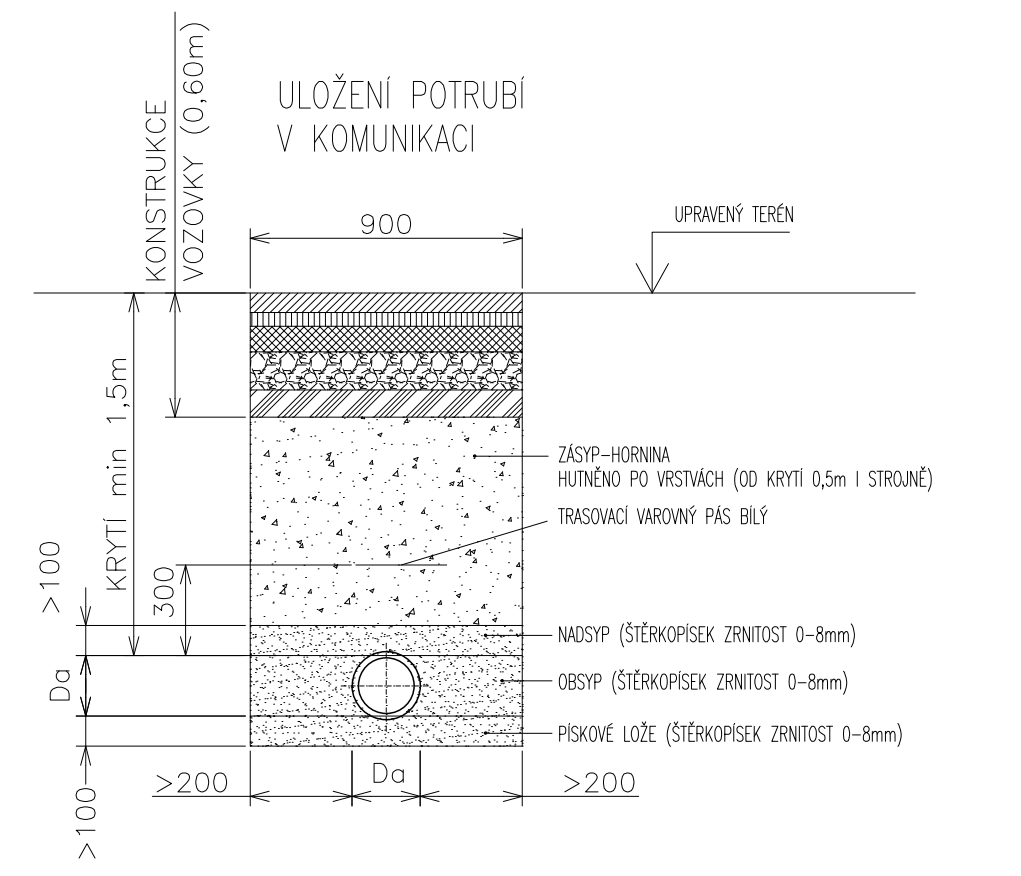
TYPICKÝ PŘÍČNÝ REZ ULOŽENÍM POTRUBÍ M1:25
