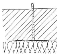
Smršťovací spára (použití kartonu)
