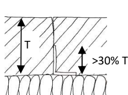
Smršťovací spára (použití L profilu)
